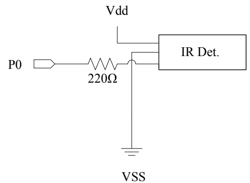
IR Detector Right
