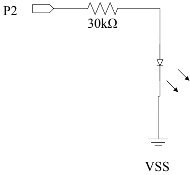
IR Emitter Right
